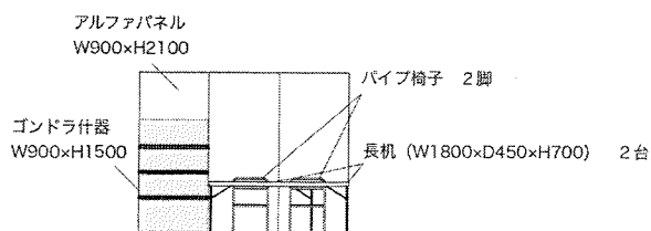
立面図（テントブース）
