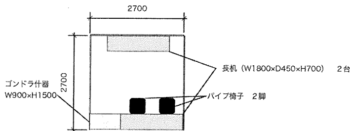
平面図（テントブース）
